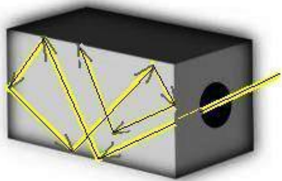
Рис. 54.2. Многократное отражение луча внутри модели приводит к его гашению
