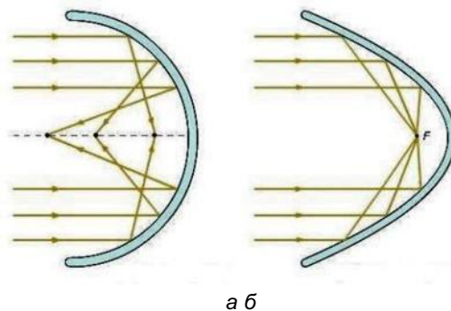
Рис. 50.7. Падающие параллельные лучи: а — в сферическом зеркале; б — в параболическом зеркале
