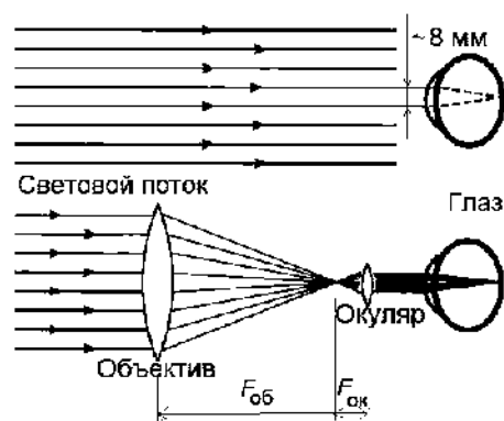
Рис. 49.4. Ход лучей в оптической системе телескопа-рефрактора
