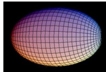
Рис. 30.6. Эллипсоид вращения
