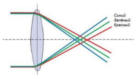
Рис. 50.5. Хроматические aberrации
