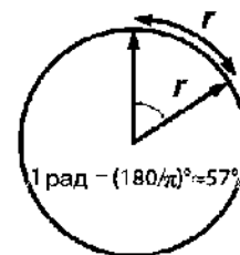
Рис. 31.2. Радиан
